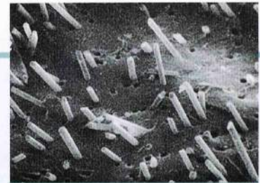
H3-material(×75) 引張り破断面(×75)
