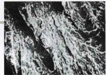
H10-material(×400) 引張り破断面(×400)
