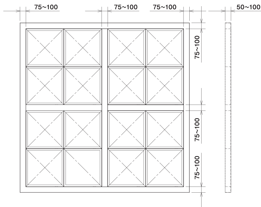
【施工例 (4段4列)】
