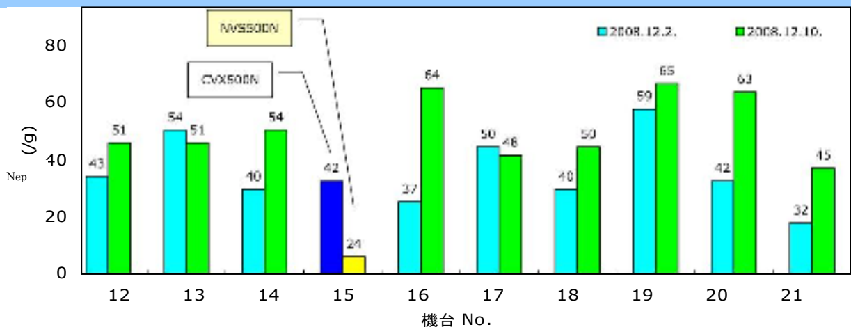
図1 DK788 Nep (USTER AFIS) (2008.12.)
